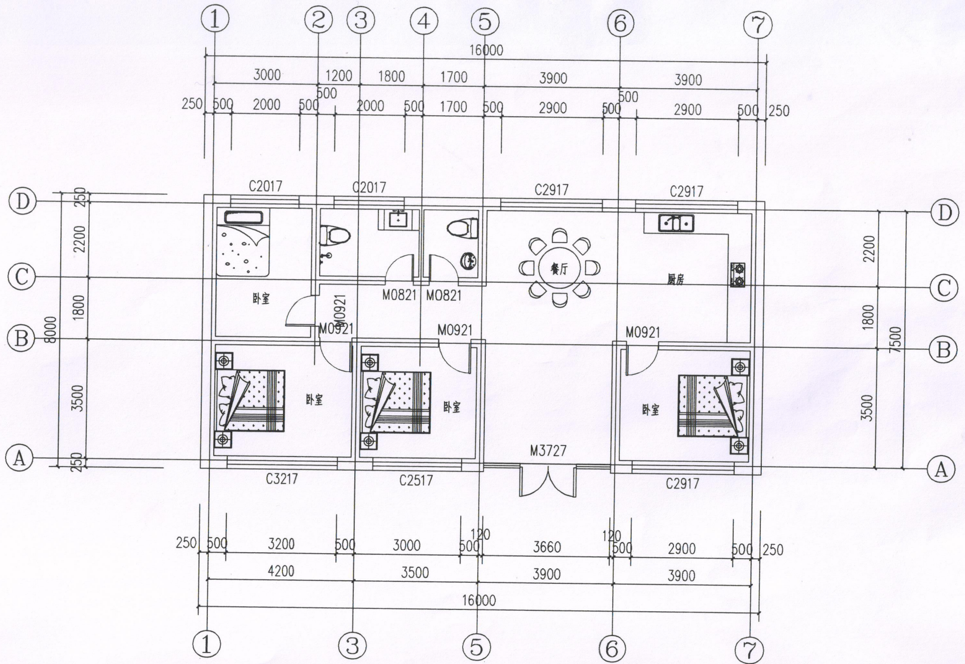
一层平面图 1: 100
